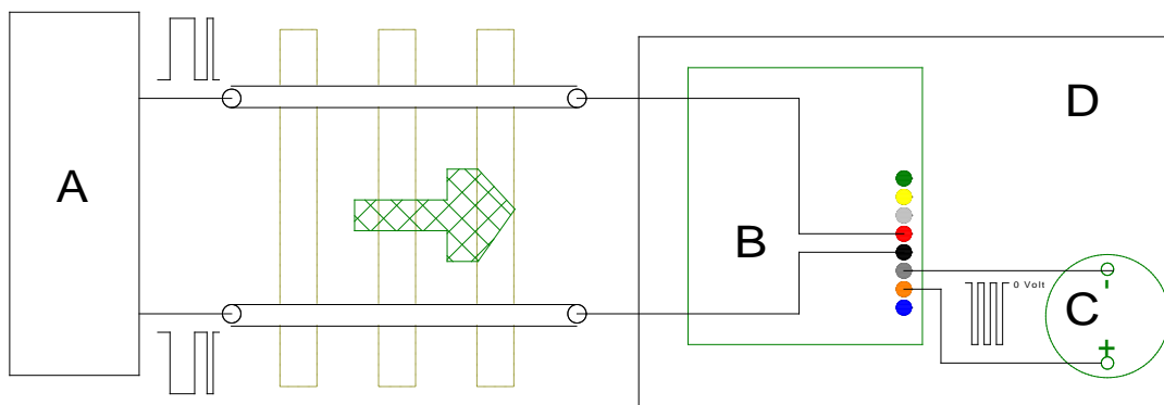
Bild 1: A = Zentrale / Booster, B = Decoder, C = DC-Motor, D = Triebfahrzeug
