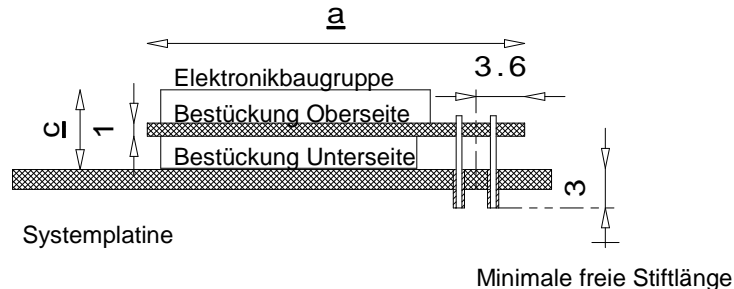
Bild 1: Anordnung des Decoders auf der Systemplatine, Maße nach Tabelle 2
