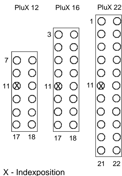
Bild 2: Zuordnung der Steckverbinder-Varianten der Ausführung PluX und Kennzeichnung der Indizierung, Ansicht auf die Buchsenleiste
