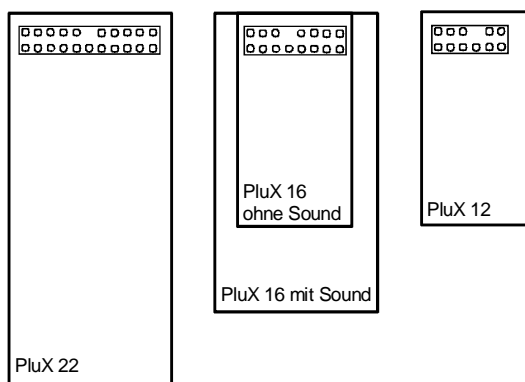
Bild 3: Größenvergleich der für die Elektronikbaugruppen reservierten Flächen abhängig von den PluX-Varianten (schematisch, etwa 1:1), Ansicht auf die Oberseite des Decoders
